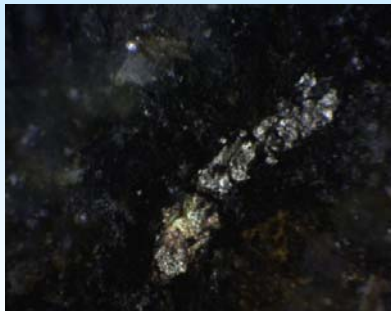
黄銅鉱(おうどうこう)
