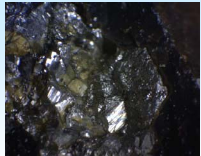
硫硫鉄鉱(りゅうひてっこう)
