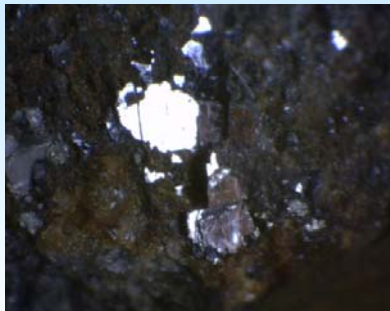
方鉛鉱(ほうえんこう)
